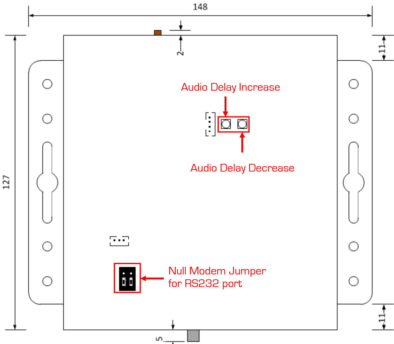
218A Bottom
