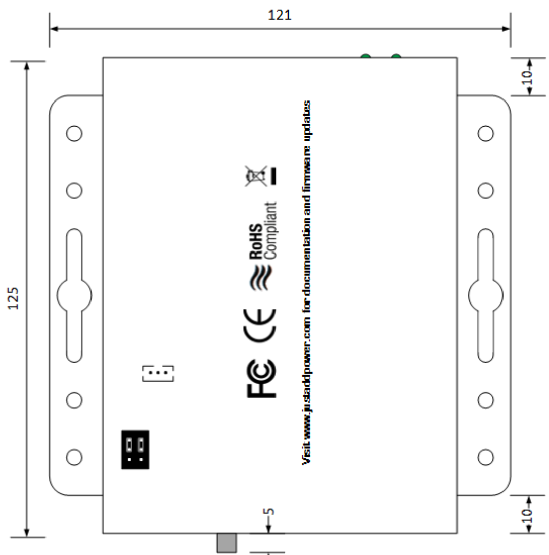
705PoE Bottom
